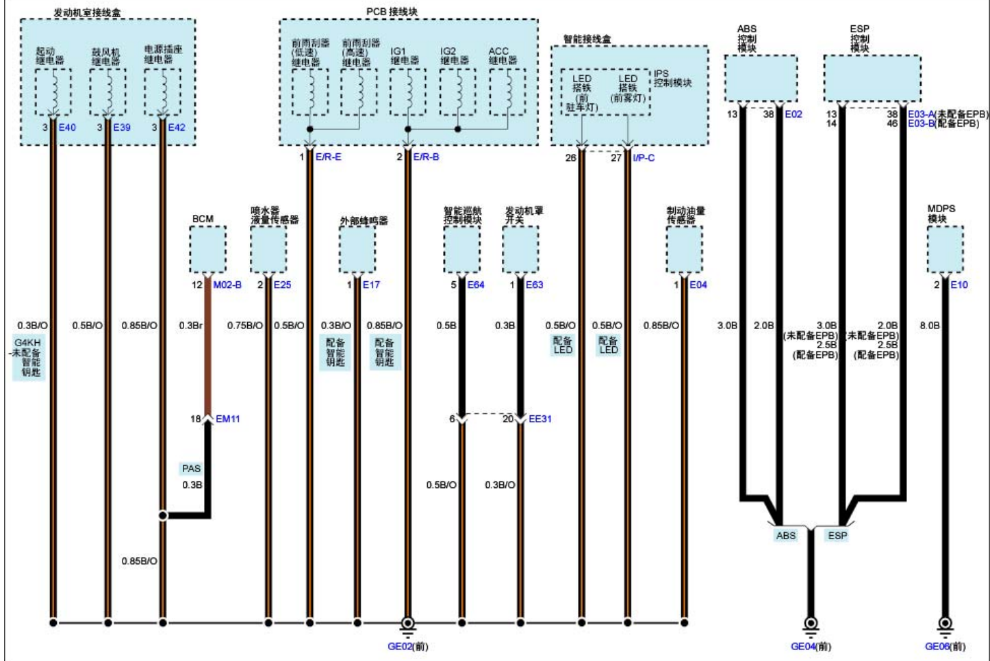
搭铁分布(6)
